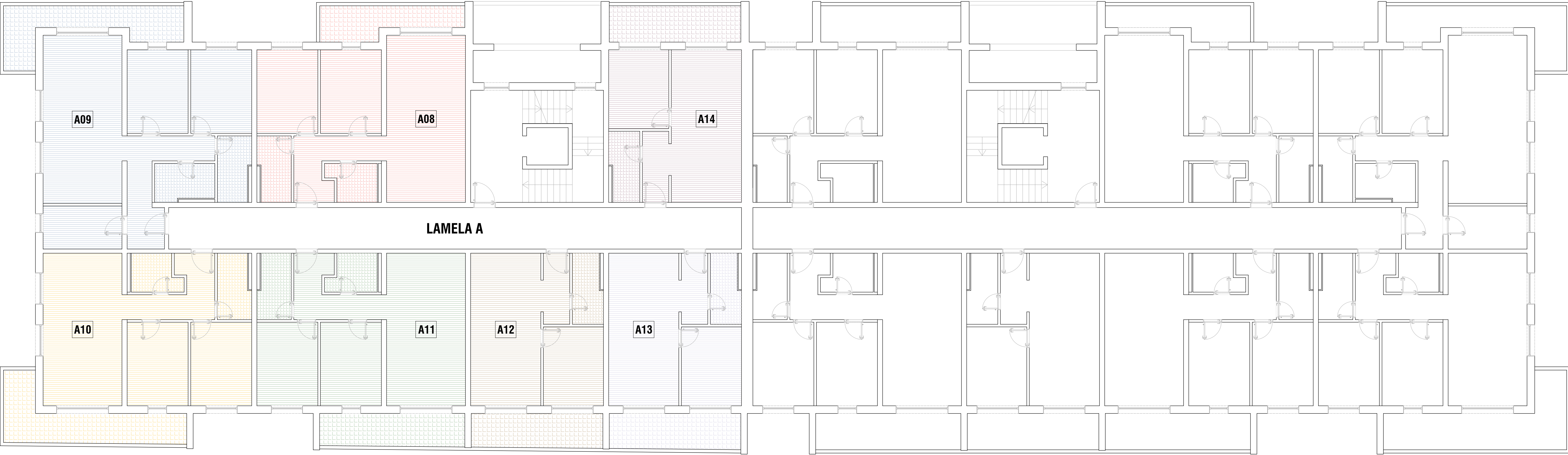
REKAPITULACIJA POVRŠINA STANOVA 2. KATA (LAMELA A)
