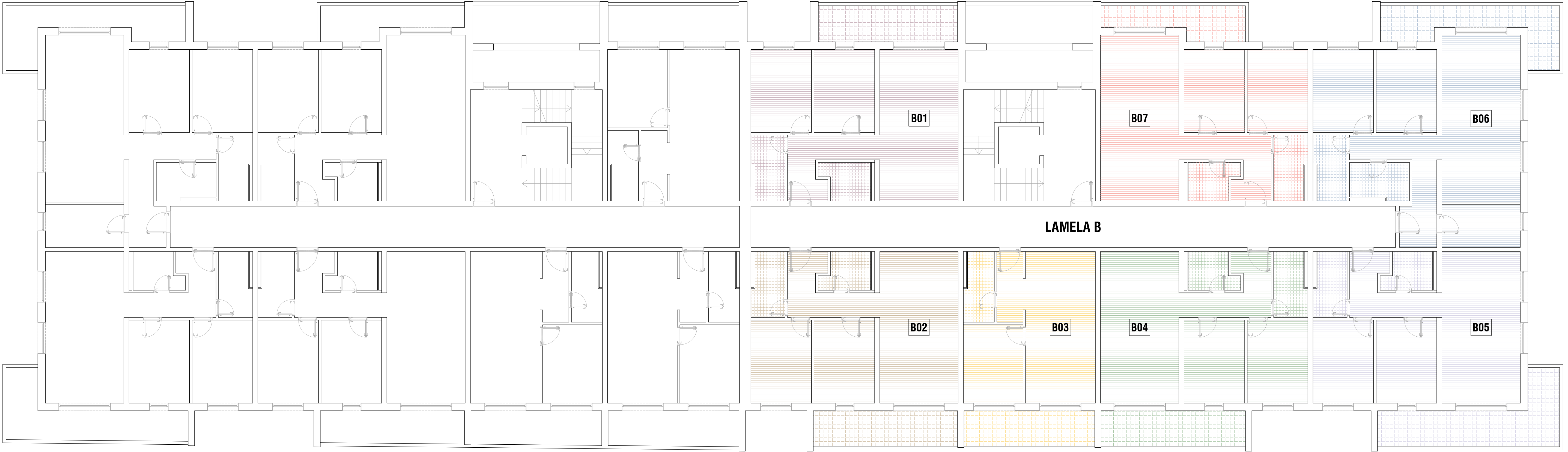
REKAPITULACIJA POVRŠINA STANOVA 1. KATA (LAMELA B)
